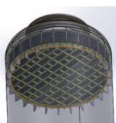
نمگیر پره ای فلزی Vane type mist eliminator
